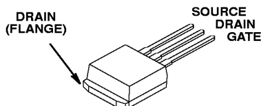
JEDEC TO-262AA
